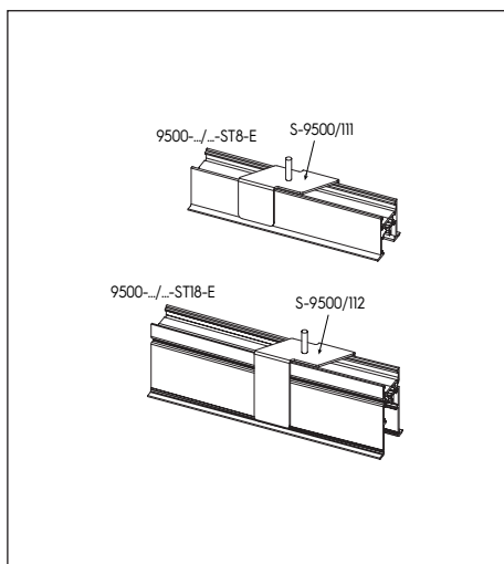
Fissaggio a clip Clip fixing
