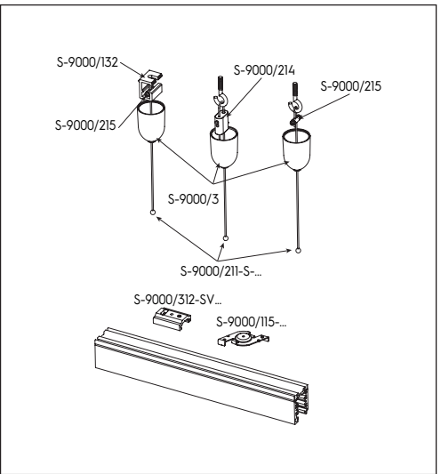
Set per fissaggio a sospensione Suspension sets
