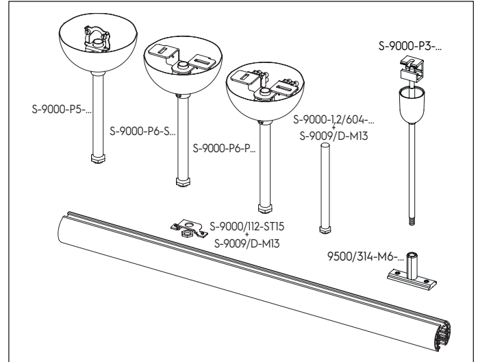
Set per fissaggio rigido a sospensione Rigid suspension sets
